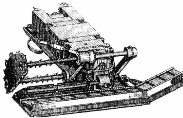
Рис. 4. Україна. Перший в світі вуглевидобувний комбайн конструкції О.І. Бахмутського
